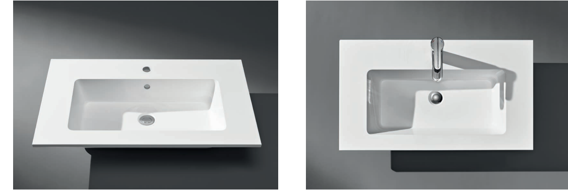
Beckenmaße: Basin dimensions // Dimensions de la vasque 605 mm: 475 x 270 mm 805 mm: 575 x 270 mm 1005 mm: 575 x 270 mm 1205 mm: 575 x 270 mm 1205 mm DWT: 475 x 270 mm
